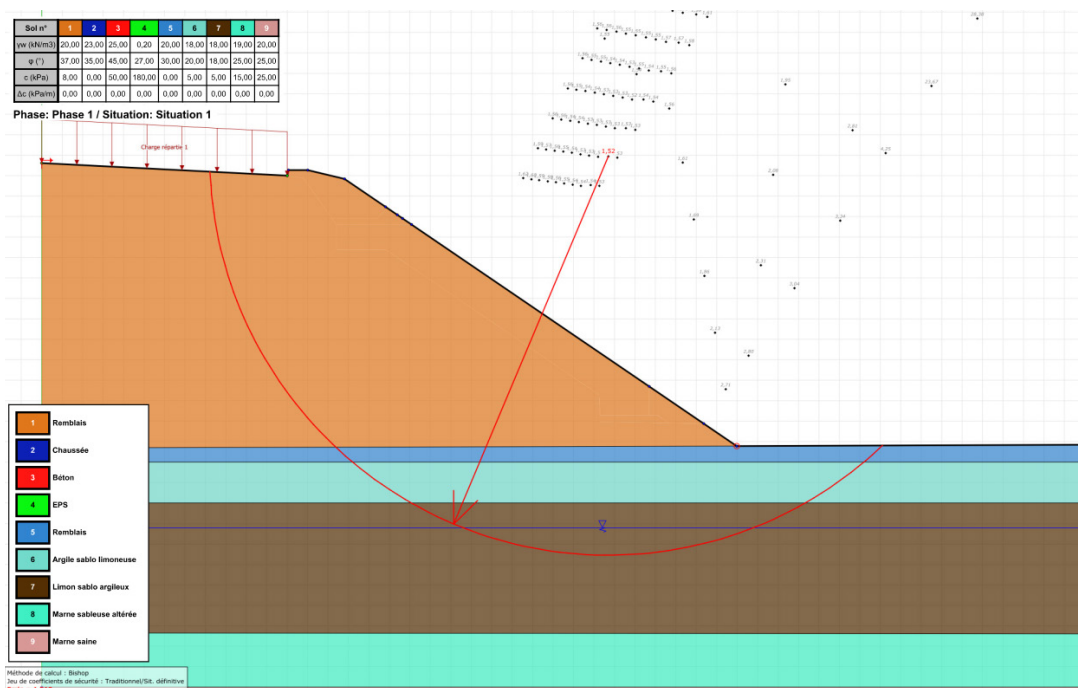
Figure 2 - Modélisation avec talus initial
