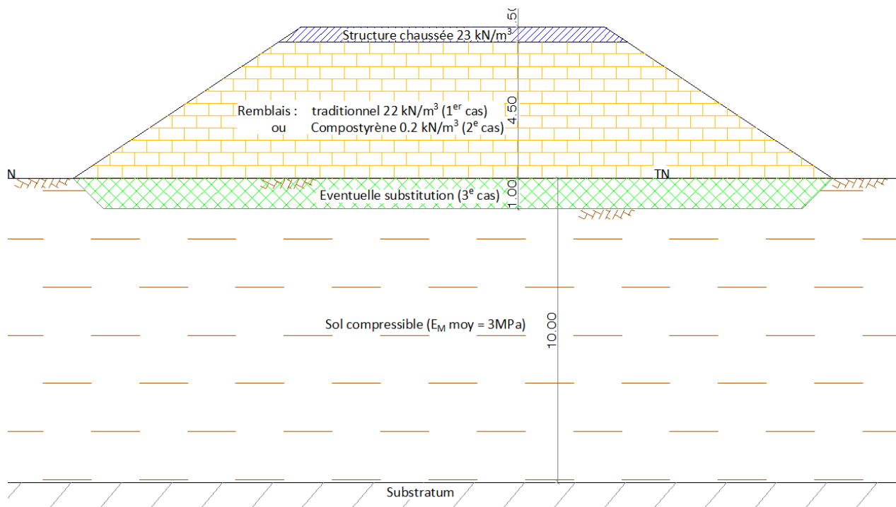
Figure 1 - Exemple de construction d'une chaussée en remblai sur sols compressibles
