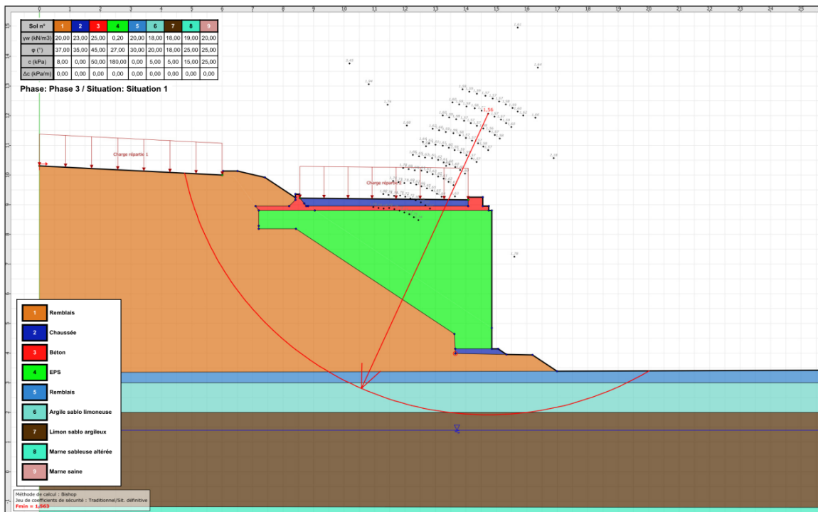
Figure 4 - Modélisation avec un remblai COMPOSTYRENE ®
