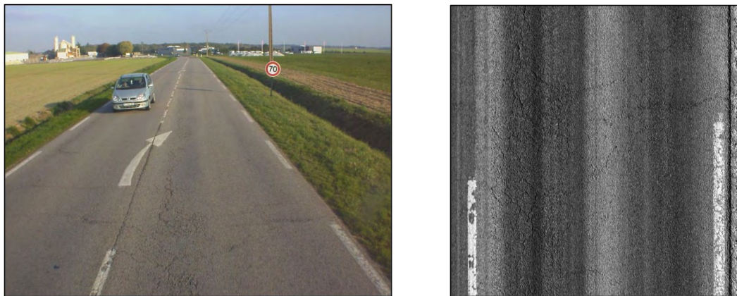
Figure 9 : Photo de dégradations (à gauche) et images LCMS de dégradations (à droite)
