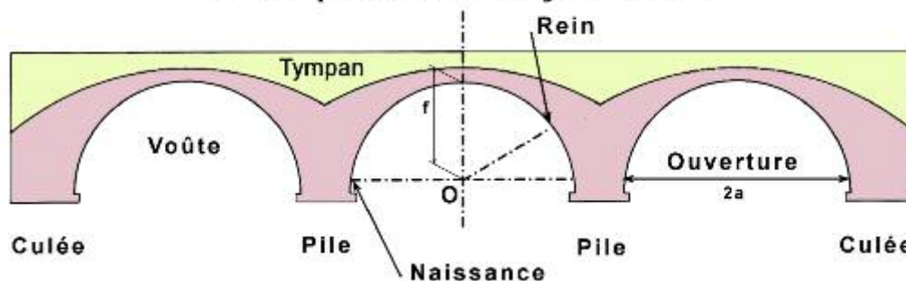
Figure n°1 : coupe longitudinale schématique d'un pont en maçonnerie
