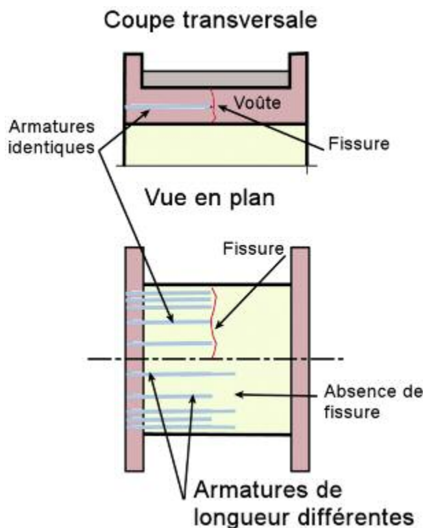
Figure n° 32 : cloutage dissymétrique
