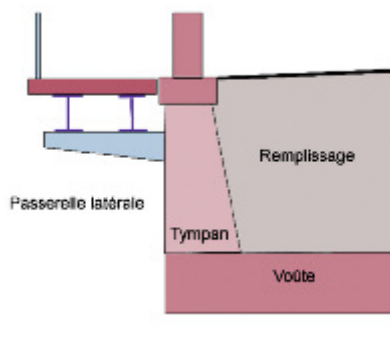
Figure n° 80 : élargissement par passerelle latérale
