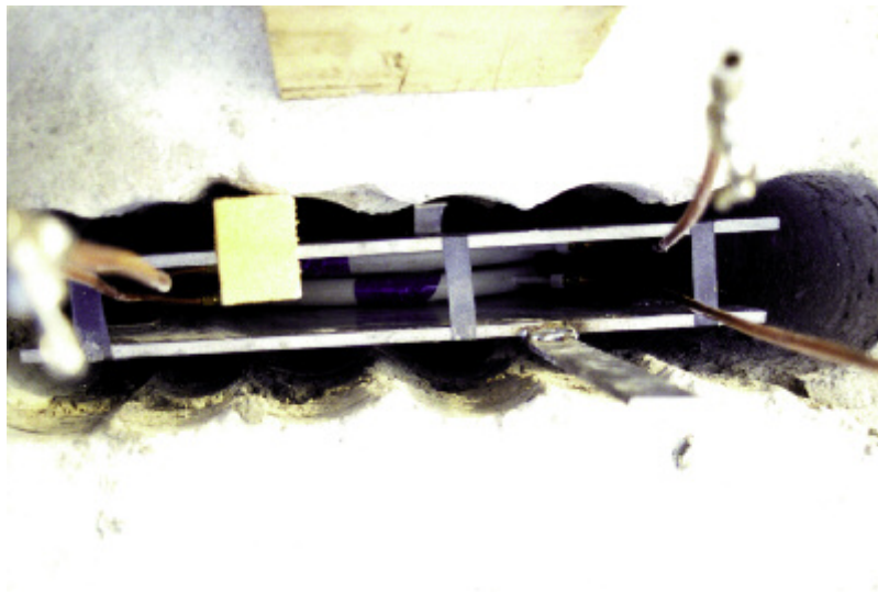
Photo n° 81 : dispositif de vérinage (crédit photo P. Vion)
