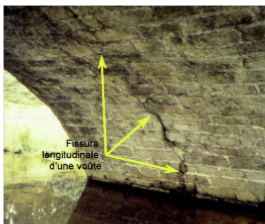
Photo n° 31 : fissure longitudinale dans une voûte (extrait IQOA - crédit photo SETRA)
