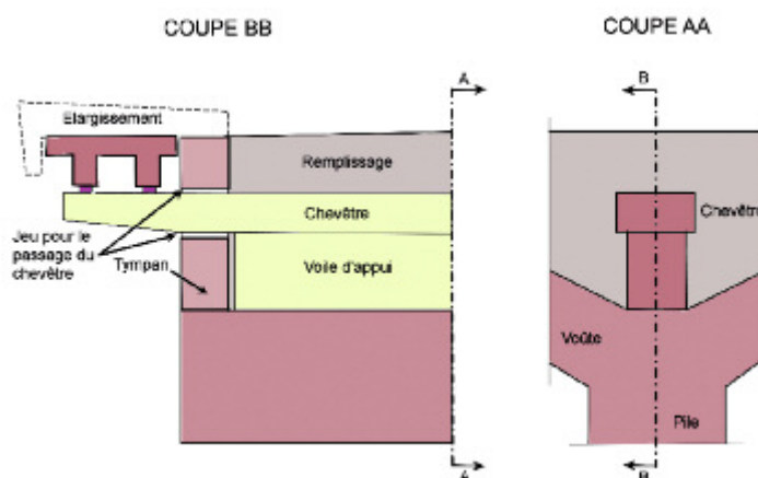
Figure n° 82 : élargissement par poutres latérales (solution 1)
