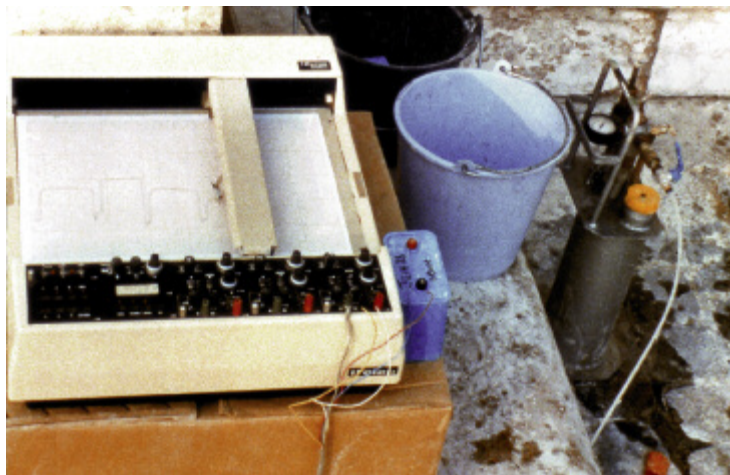
Photo n° 26 enregistreur XY (crédit photo A. Bouineau)
