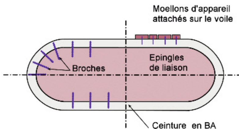
Figure n° 66 : ceinturage de protection d'une pile en maçonnerie
