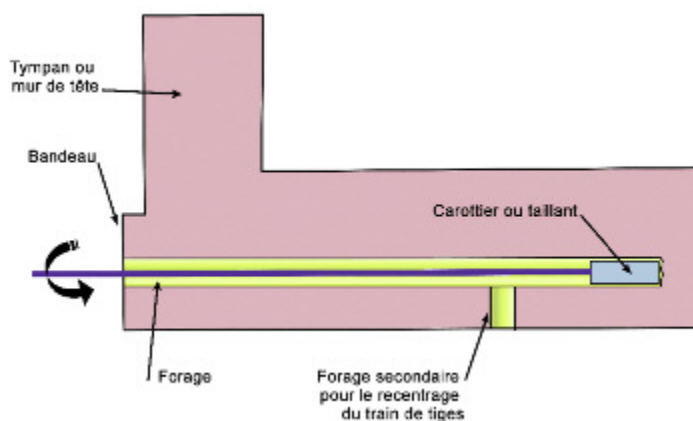
Figure n° 50 : principe à appliquer pour centrer le forage
