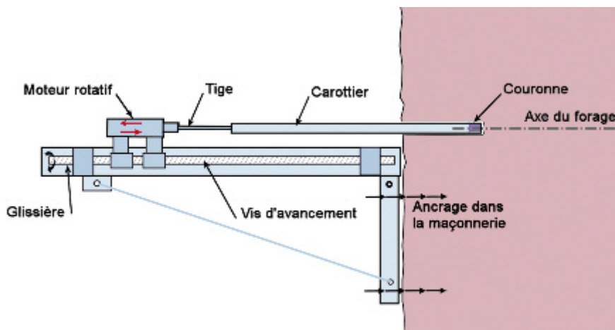
Figure n° 47 : schéma d'un forage au carottier
