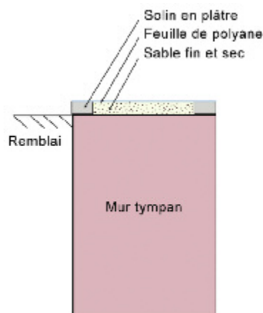
Figure n° 77 : boîte à sable
