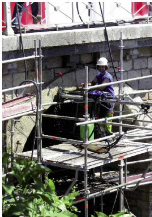
Photo n° 59 : forage du bandeau et de la voûte au pont des Abarines (crédit photo Cofex Littoral)
