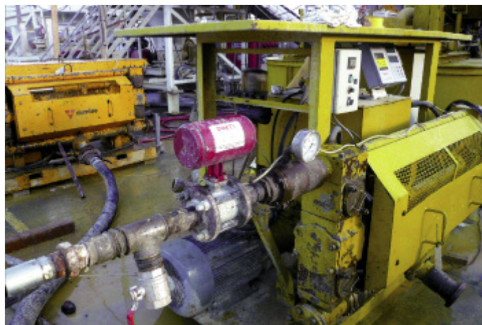
Photo n° 24 : détail d'un dispositif de mesure de la pression et du débit d'injection (crédit photo DIMTI)
