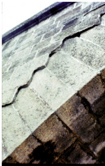
Photo n° 32 : décollement entre le tympan et le bandeau du pont du nid d'oise à Clisson (crédit photo CETE de l'Ouest - Jacques Billon)
