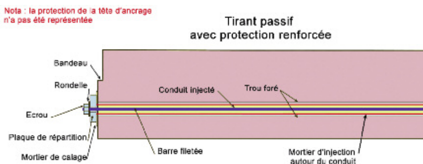
Figure n° 51 : tirant d'enserrement avec protection renforcée
