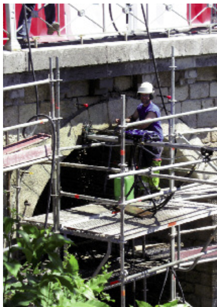
Photo n° 49 : forage dans le corps de voûte marteau hors trou (crédit photo Cofex Littoral)
