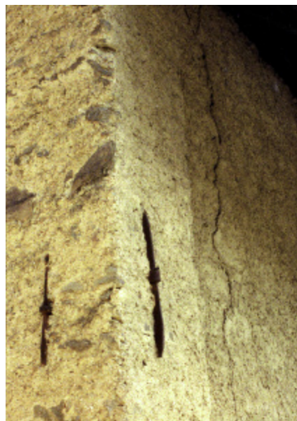
Photo n° 36 : tirants d'enserrement d'un bâtiment dans les Hautes-Alpes (crédit photo D. Poinéau)
