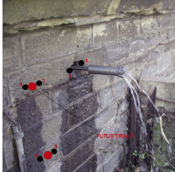
Photo n° 50 : sortie du taillant (crédit photo Cofex Littoral)
