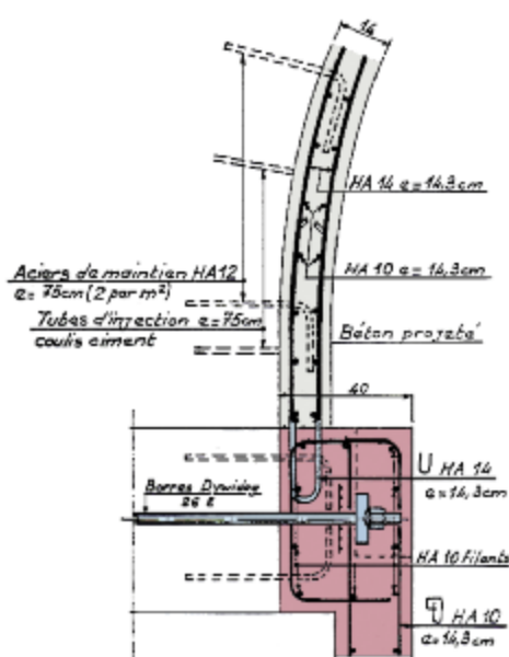
Figure n° 65 : exemple de ferrailage d'une contre-voûte (document fourni par J.L. Michotey)
