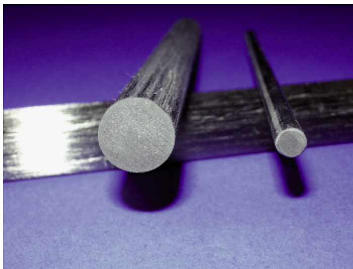
Photo n° 47 : armatures en composites pour béton armé (crédit photo Freyssinet)
