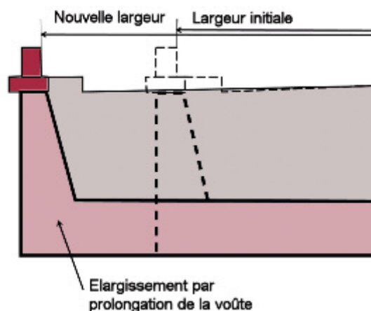
Figure n° 86 : élargissement par prolongation de la voûte
