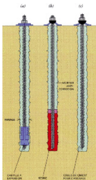
Figure n° 35 : les trois sortes de boulons d'ancrage (d'après la documentation DSI France)
