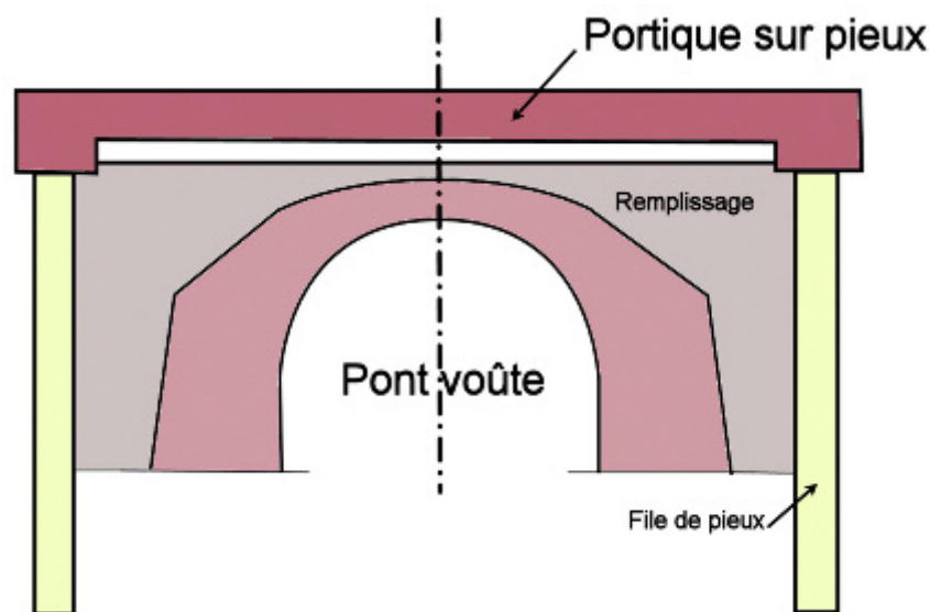
Figure n° 87 : élargissement de type pontage
