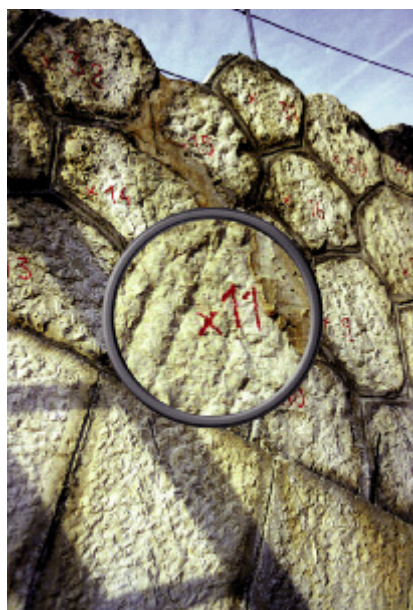
Photo n° 4 : repérage des moellons des tympons du pont de Villeneuve-Loubet avant leur démontage (crédit photo P. Vion)
