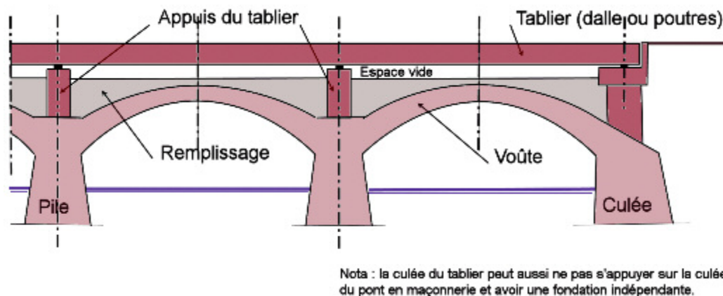
Figure n° 83 : élargissement par un tablier de toute largeur reposant sur les appuis de l'ouvrage en maçonnerie
