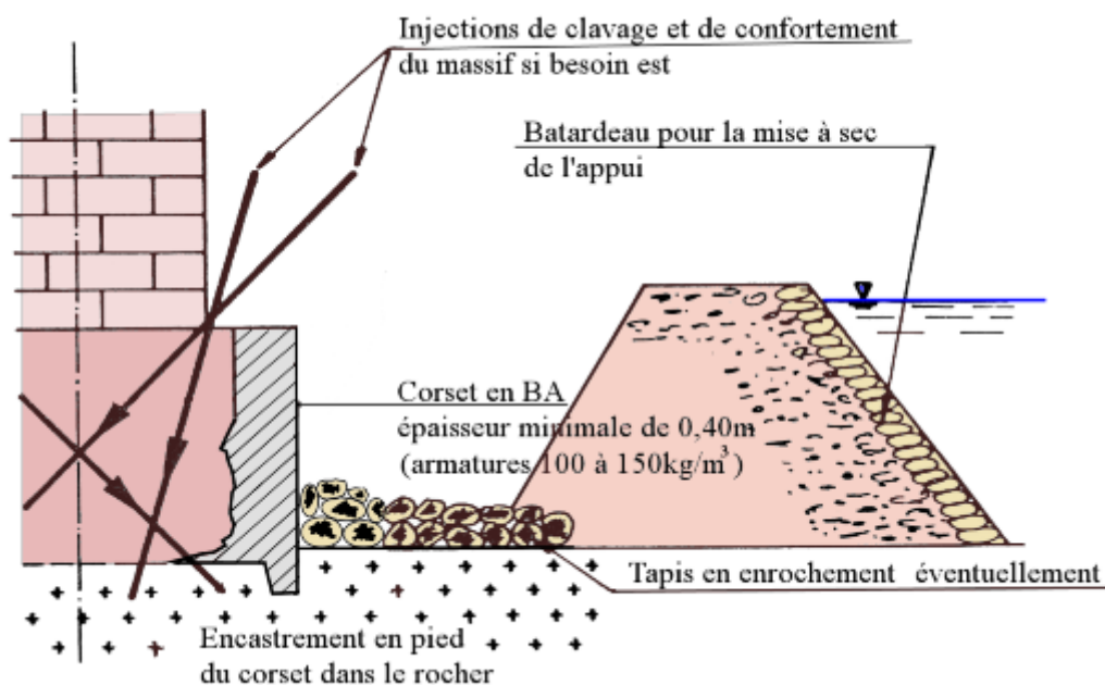
Figure n° 23 : exemple d'un massif de béton de chaux désorganisé conforté par un corset en béton armé et une injection de régénération du liant
