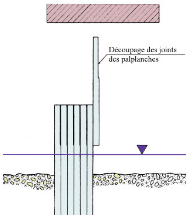
Figure n° 21 : découpage des joints
