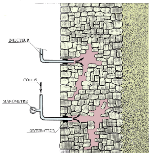
Figure n° 25 : injection à l'avancement par passe descendante
