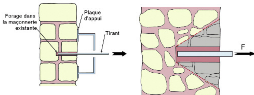
Figure n° 30 : principe de l'essai d'ancrage
