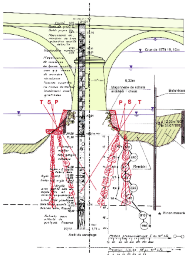
Figure n° 28 : réalisation d'une injection solide de renforcement de la portance d'une fondation du pont de Verdun à ANGERS
