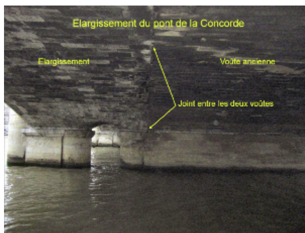
Photo n° 93 : élargissement du pont de la Concorde entre 1930 et 1932 (crédit photo D. Poineau)
