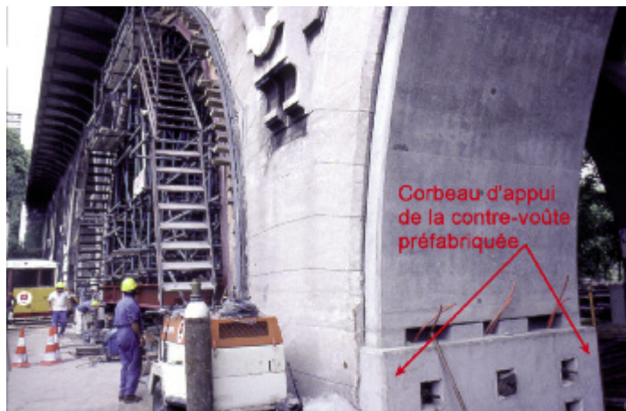
Photo n° 70 : longrine d'appui en partie basse de la contre-voûte préfabriquée du pont de Levallois (crédit-photo D. Poinneau)
