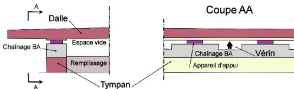
Figure n° 78 : solution variante d'élargissement par dalle générale
