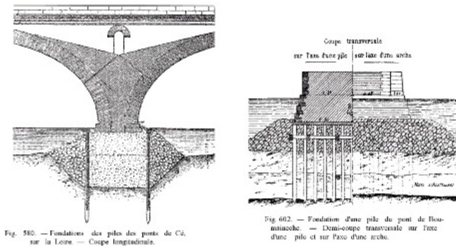
Figure n° 5 : protection de fondations anciennes par des talus d'enrochement (extrait du tome II du traité des ponts en maçonnerie et tunnels de J ; Chaix et Chambaret Éditeur : Fanchon et Artus [Paris] vers 1889)
