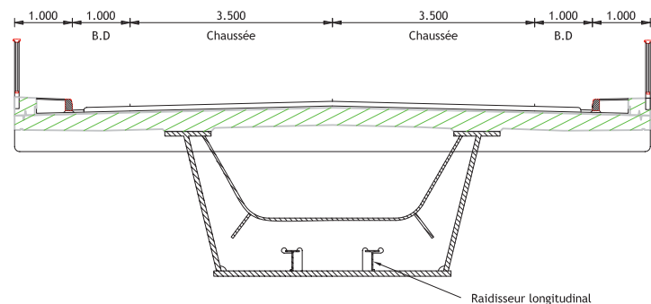
Caisson à pièces de pont
