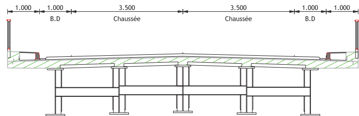
Multipoutre à entretoises
