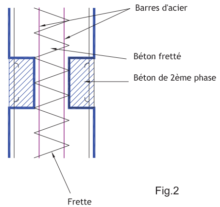
Articulation CONSIDERE (début du 20 e siècle)
