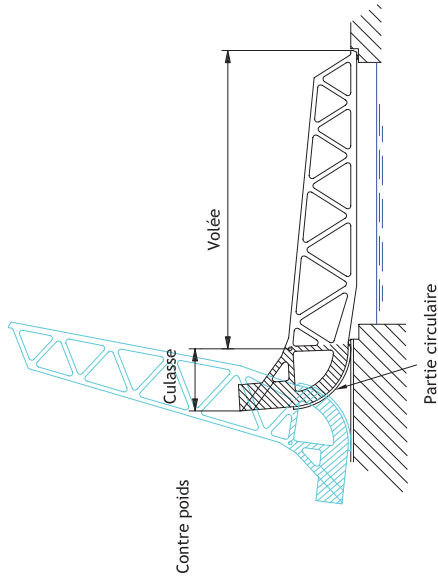
Pont basculant
