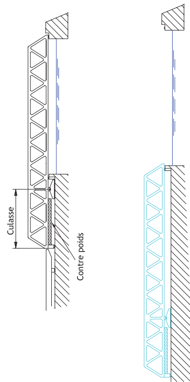
Pont rétractable
