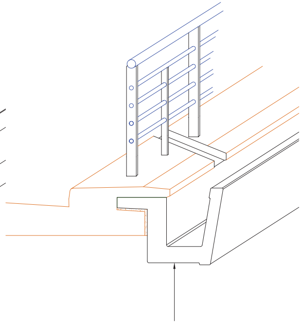
Fig.2 Corniche caniveau béton
