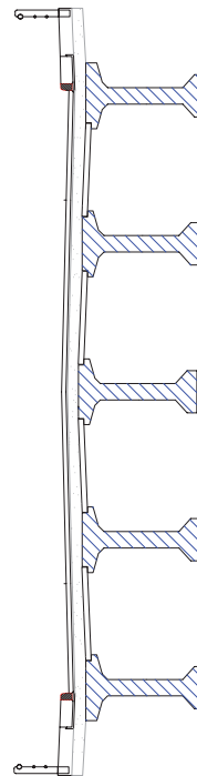
(V.I.P.P) Viaducs à travées indépendantes à poutres préfabriquées précontrainte par post-tension
