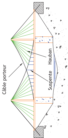
Pont Gisclard
